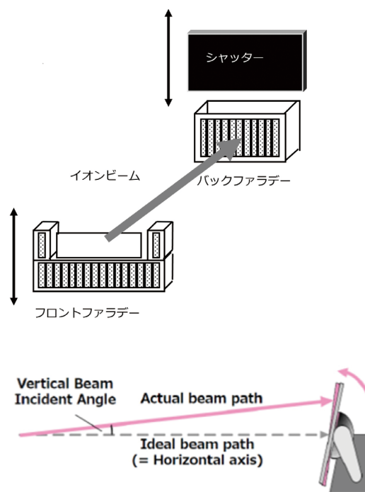
図2 イオン計測と角度補正システム
