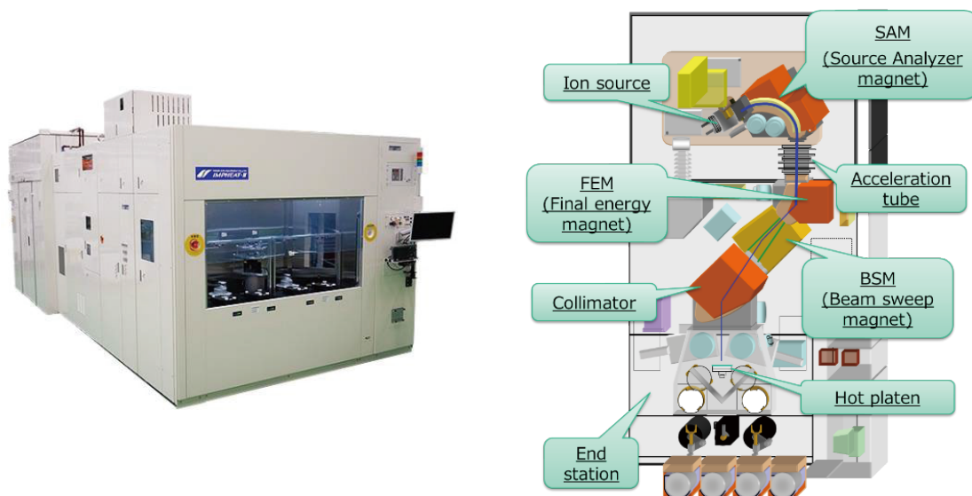
図1 「IMPHEAT」の外観および概略
