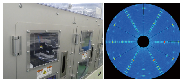
図3 XRD 装置搭載状態とXRD測定結果
