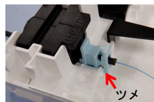
③ツメが引かかる（カチッと音がする）までから押し込む
