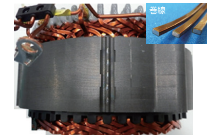
環境対応車用モーター平角巻線
