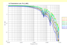
挿入損失
