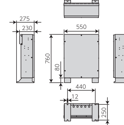
【本体寸法図】
