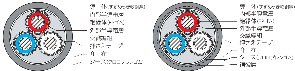
高圧2PNCT
