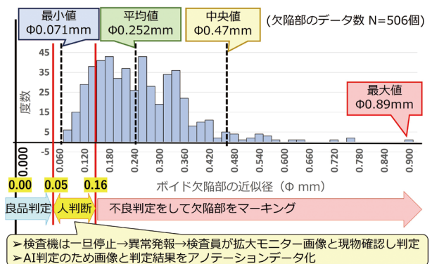
図3 欠陥部の画像処理検査判定方法
