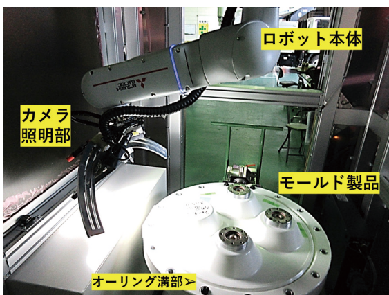
写真1 モールド部品用外観自動検査ロボット
