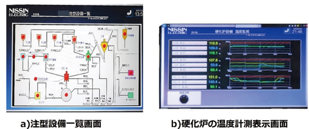
図5 注型設備と硬化炉のIoTデータ表示画面
