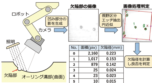
図4 撮像方法の概念図と画像処理判定の事例
