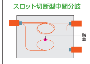
写真はMJC-FNB3 ※実装例・製品にはケーブル・コード類は含まれません。
