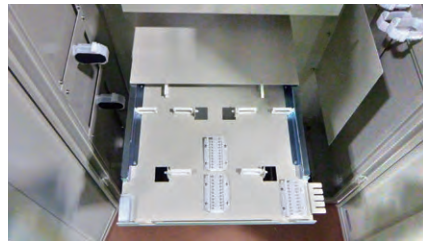
40接続融着トレイ
