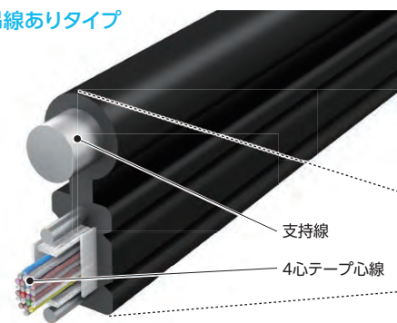
吊線ありタイプ
