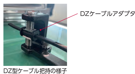
DZ型ケーブル把持の様子
