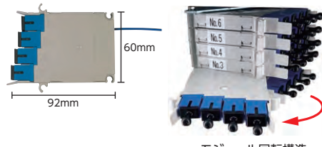
モジュール回転構造
