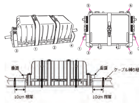
ガスケットは内側に倒れたり、スリーブで挟み込んだりしないよう注意して取り付けます。
