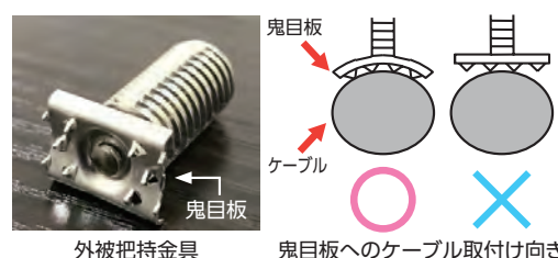
外被把持金具 鬼目板へのケーブル取り付け向き
