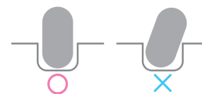
ガスケットは内側に倒れたり、スリーブで挟み込んだりしないよう注意して取り付けます。
