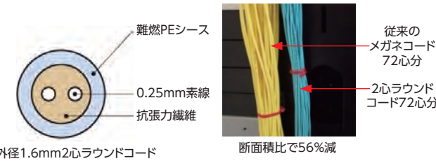
外径1.6mm2心ラウンドコード
