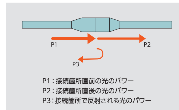
光コネクタの接続箇所の模式図
