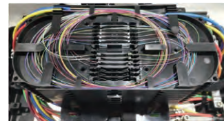
融着接続トレイ
