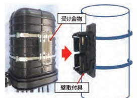
ポールマウント (MJC-GP8の例)
