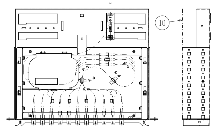
*上図は「Y-OP4-FD<48C-2U><SC><P2><44C><F>」を示す。
