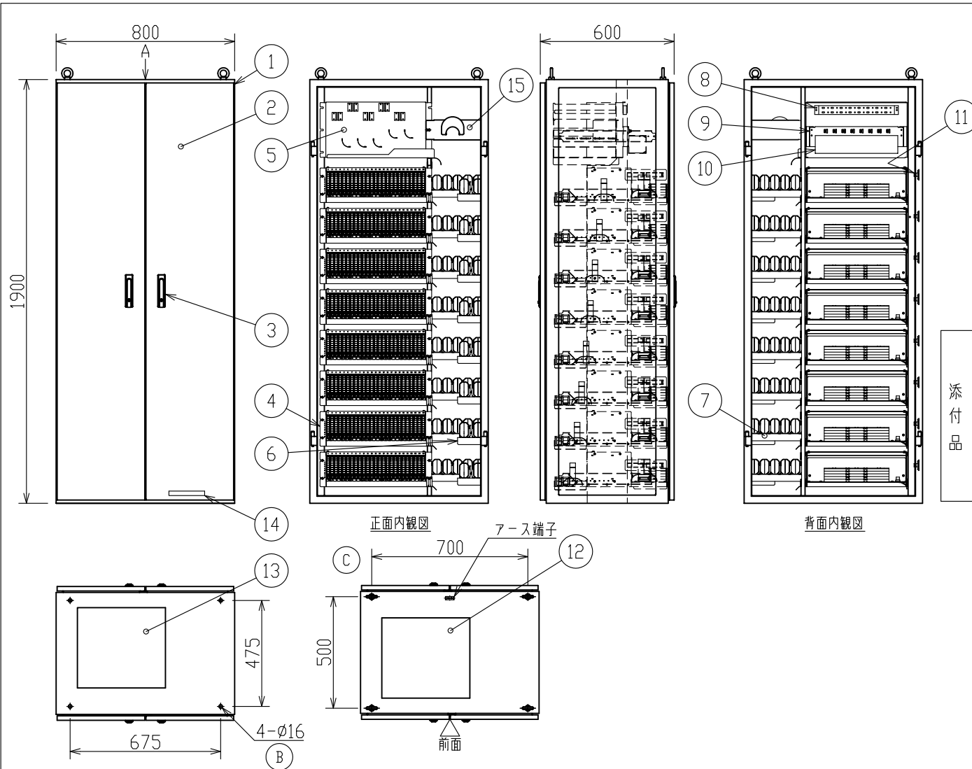
矢視 A
