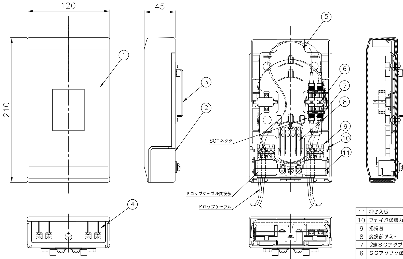
内部構造及び配線図
