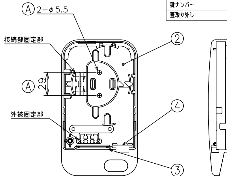
内部構造（正面／側面）
