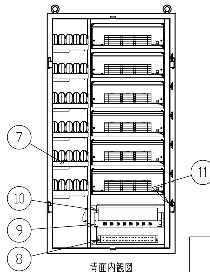
背面内観図
