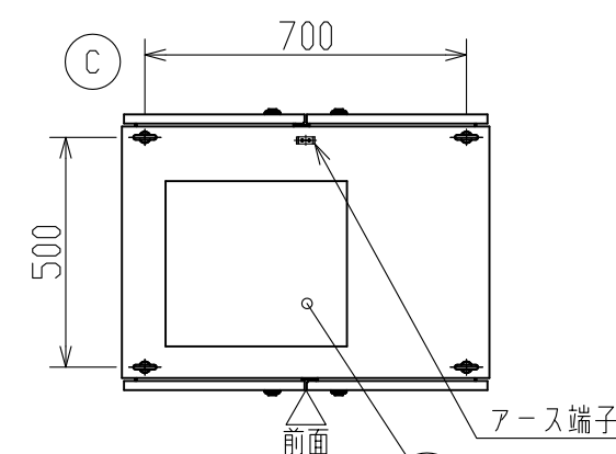
矢視 A
