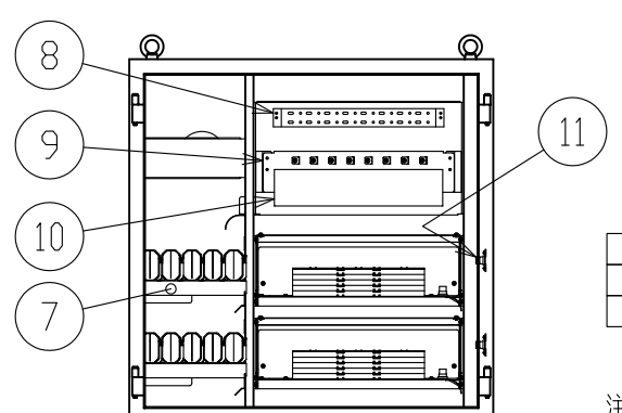
背面内観図
