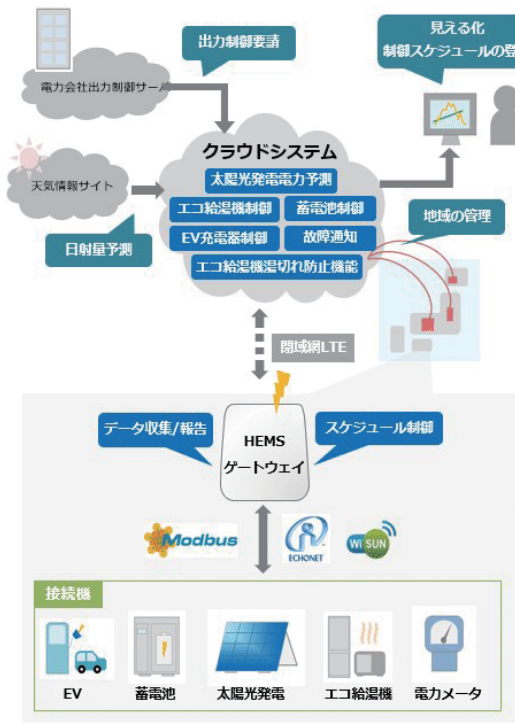
図2 SPSS-Hシステム構成
