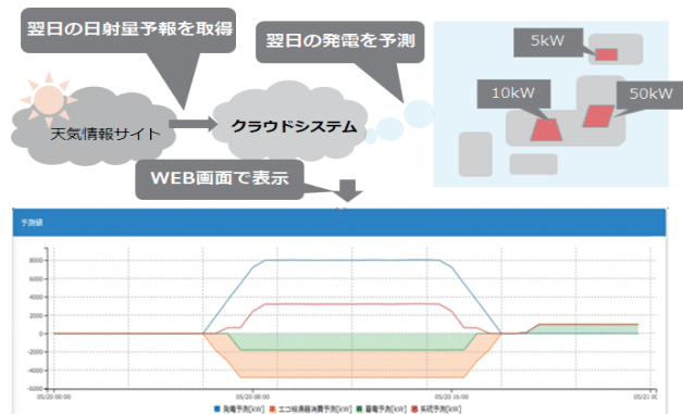
図3 太陽光発電電力予測
