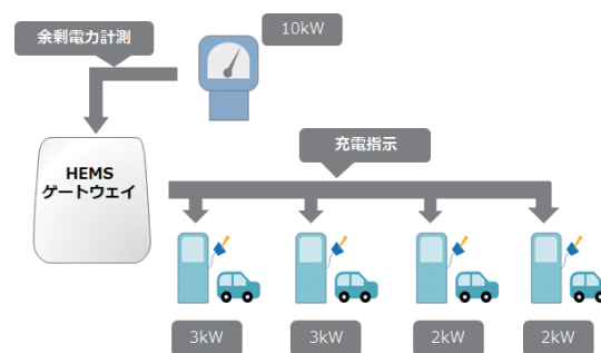
図6 EV充電器制御
