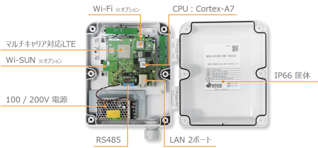
写真2 HEMSゲートウェイ
