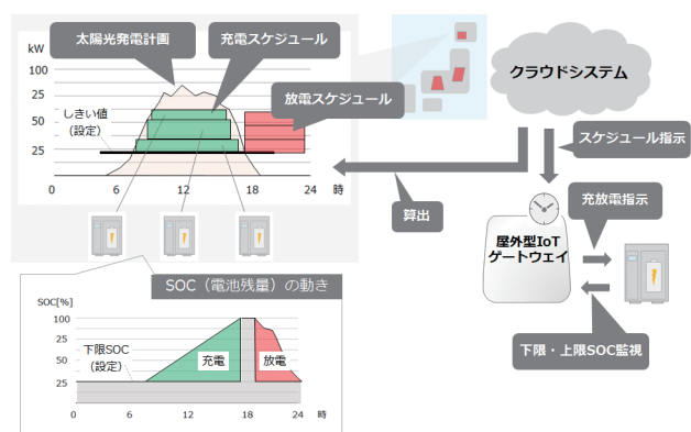
図4 蓄電池制御
