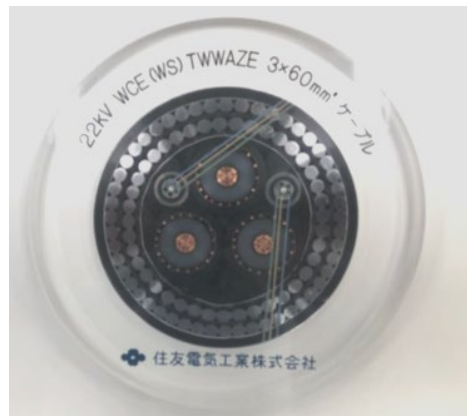
写真1 ダイナミックケーブル
