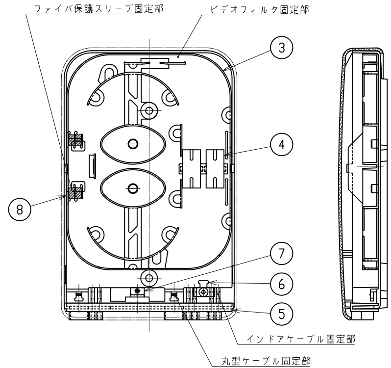
内部構造
