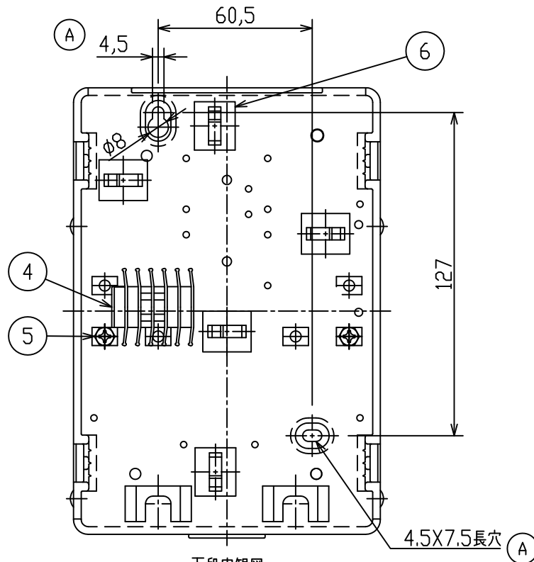
下段内観図
