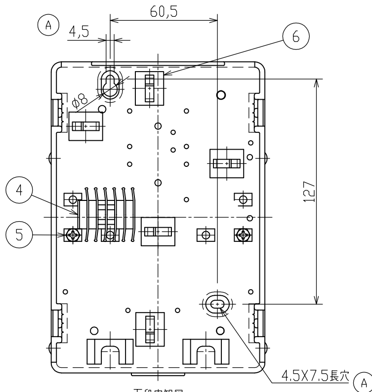
下段内観図
