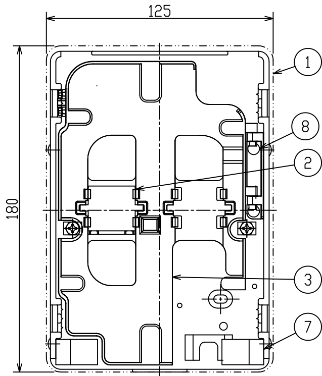
上段内観図
